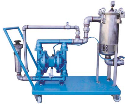
Ligne de transvasement avec pompe à membranes en aluminium-téflon de 1 1/2" et deux filtres cunos courts (10")
