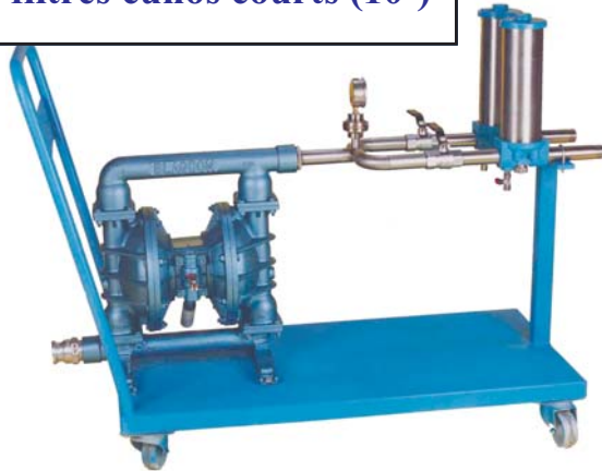
Ligne de transvasement avec pompe à membranes en aluminium-téflon de 1 1/2" et deux filtres cunos courts (10")
