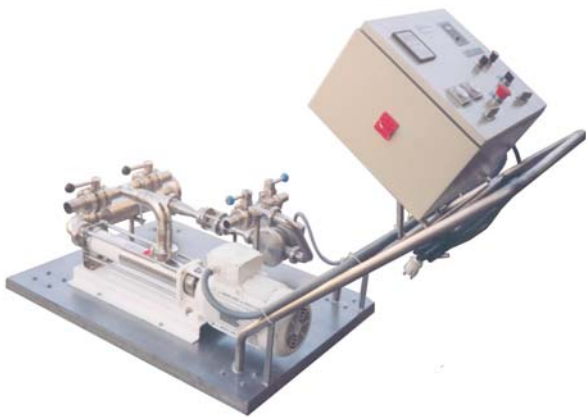
Ligne de dosage avec pompe genre mono avec compteur à roue ovale et un programmeur
