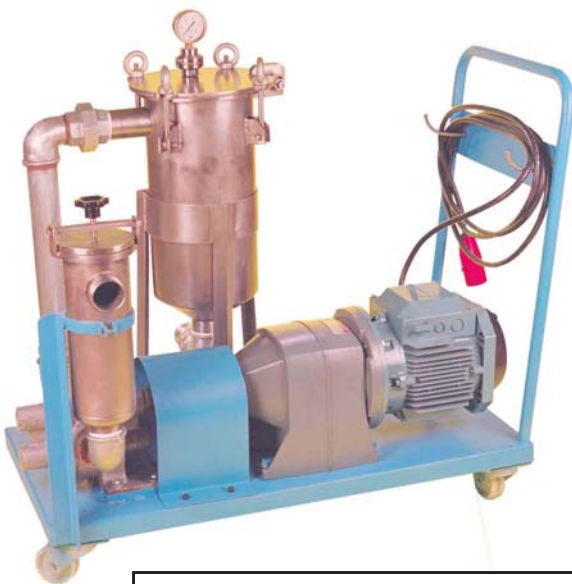
Pompe d'engrenages avec pré-filtre de 2" et poches filtrantes de 2"
