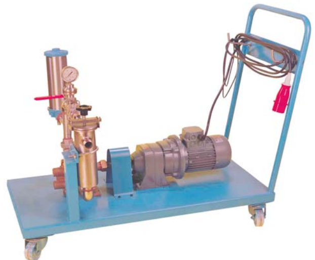
Pompe d'engrenages avec pré-filtre de 1" et un filtre cuno court (10")
